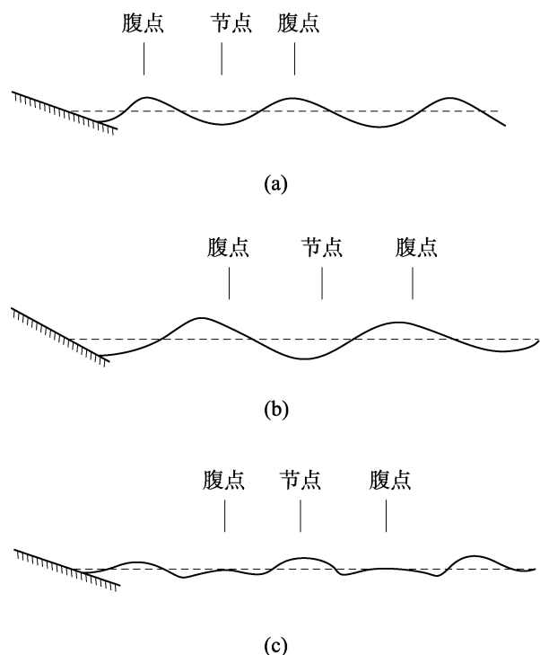
图 D.0.1 斜坡堤前的 3 种冲刷形态示意图
