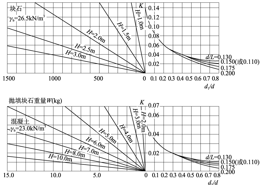
图 E.0.1 明基床基肩和坡面块体稳定重量计算图
