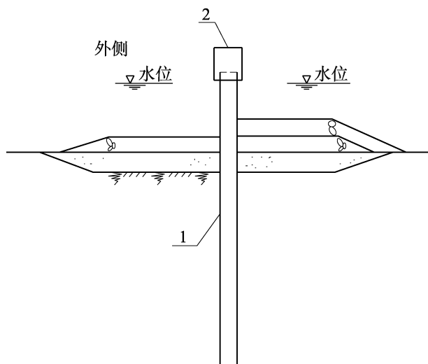
图 5.8.1 单排桩直立堤断面型式
