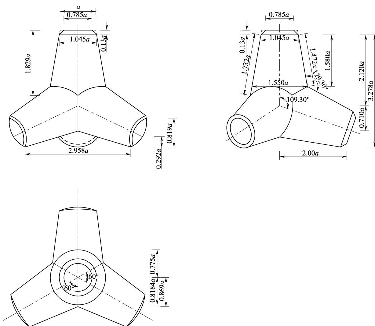
图 B.0.1-1 四脚锥体 a -四角锥体基准尺寸
