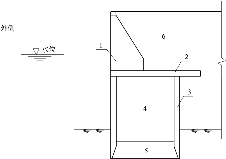
图 8.2.7 沉井式护岸结构断面型式
