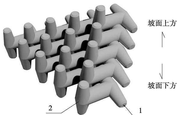
图 4.4.5-2 扭工字块体规则安放示意图
