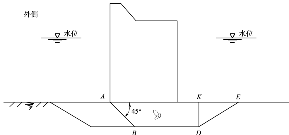
图 5.3.9-2 暗基床滑动面示意图
