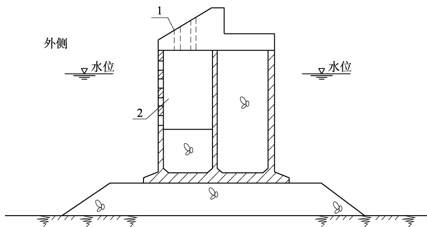
图 5.6.1 开孔沉箱直立堤断面型式
