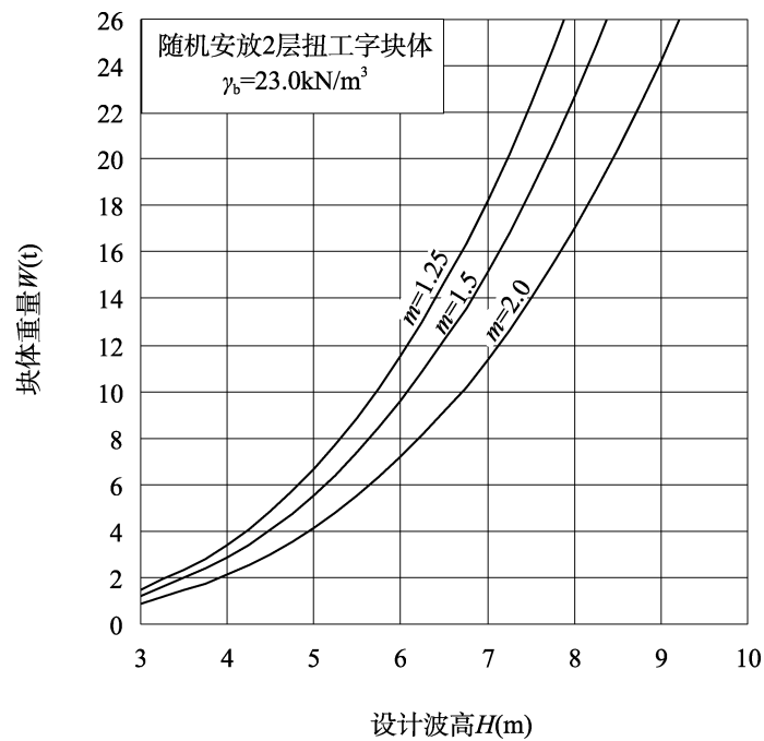
图 C.0.4-1 扭工字块体的稳定重量 W ( K_D = 18 )
