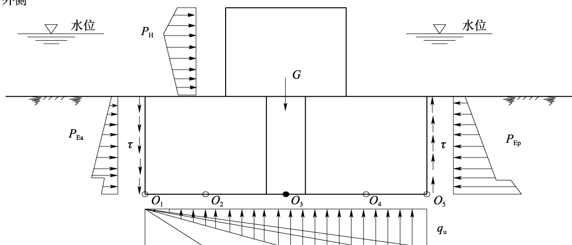
图 K.0.5 箱筒型基础结构防波堤抗倾稳定性计算简图
