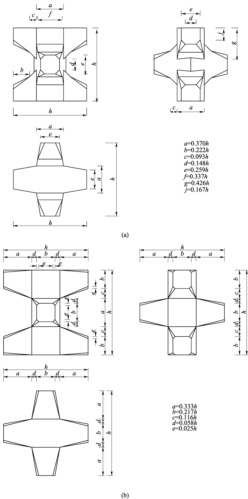
图 B.0.1-4 扭王字块体
