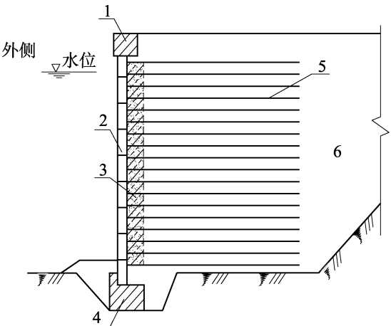
图 8.2.4 加筋土岸壁断面型式 1-胸墙或帽梁;2-墙面板;3-倒滤层;4-基础;5-加筋体;6-回填料
