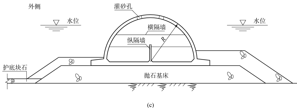
图 6.2.1 半圆型防波堤的断面型式
