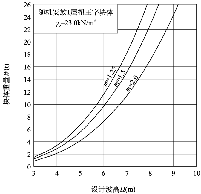
图 C.0.5-1 扭王字块体的稳定重量 W(K_D = 18)
