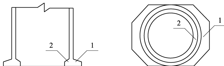
图 5.7.6 圆筒底部加强图
