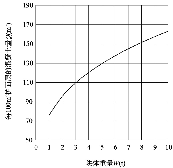
图 C.0.2-3 四脚锥体的混凝土量 Q
