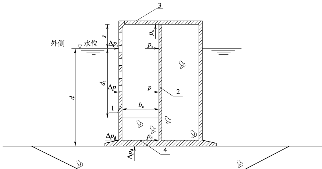
图 H.0.4 波峰作用时,有顶板开孔矩形沉箱结构上的波压力和压差
