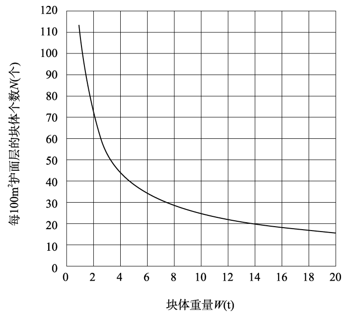
图 C.0.5-2 扭王字块体的个数 N (随机安放 1 层)
