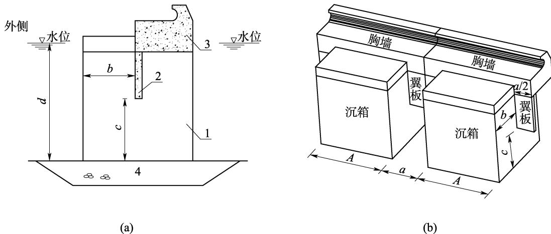
图 6.3.5 沉箱墩式透空堤断面型式
