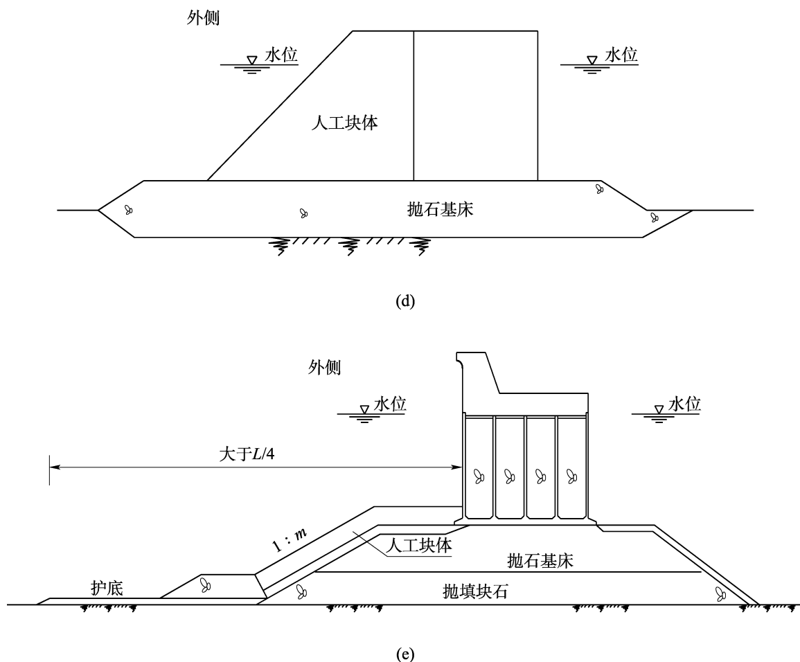
图 5.2.1 重力式直立堤断面型式
