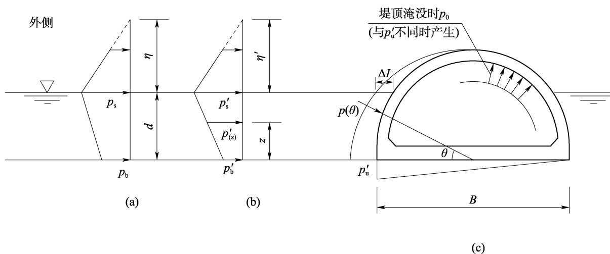
图 J.0.1 半圆型堤上的波压力分布图
