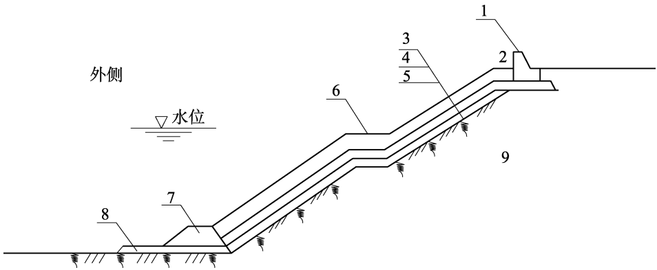
图 7.2.1-2 坡式护岸断面型式
