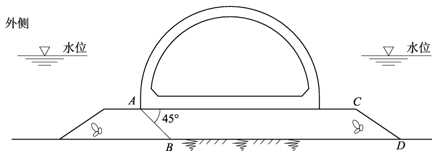
图 6.2.3-1 明基床滑动面示意图
