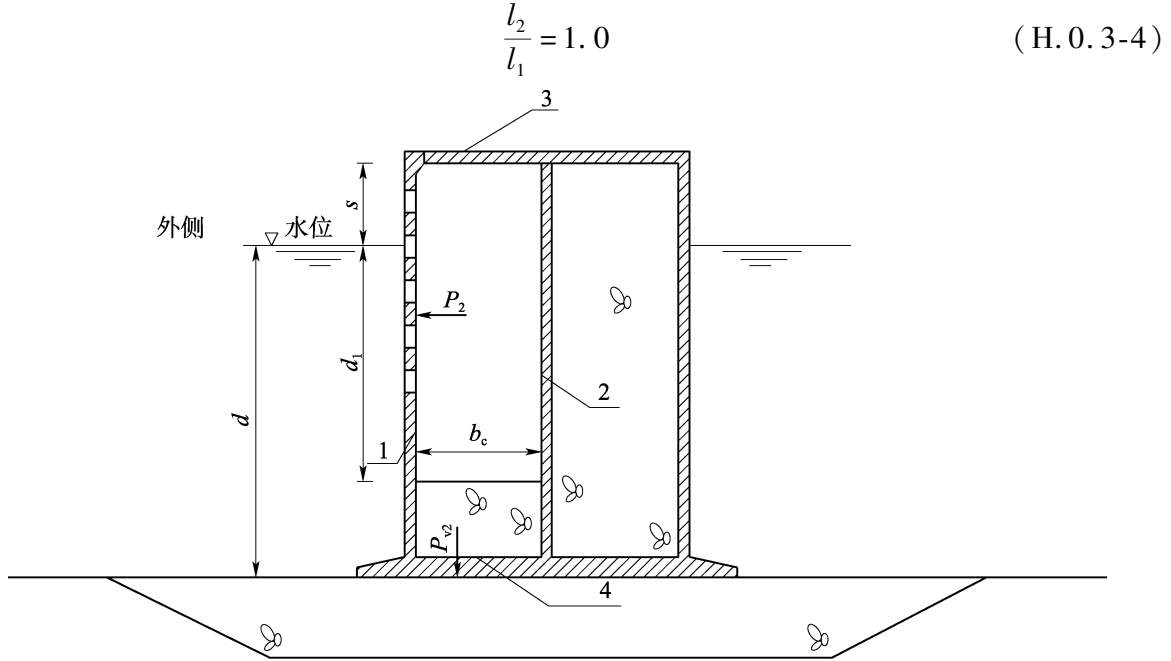
图 H.0.3 波谷作用时,有顶板开孔矩形沉箱结构上的波浪力
