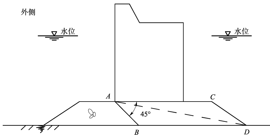
图 5.3.9-1 明基床滑动面示意图
