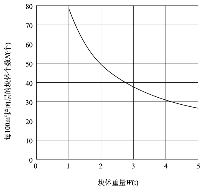
图 C.0.3-2 四脚空心方块块体个数 N
