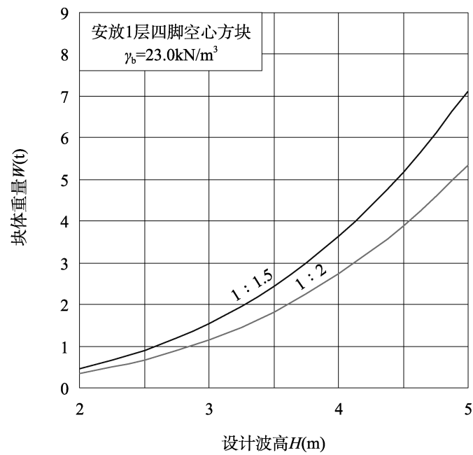
图 C.0.3-1 四脚空心方块的稳定重量 W
