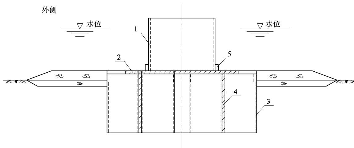
图 6.4.1 箱筒型基础防波堤断面型式
