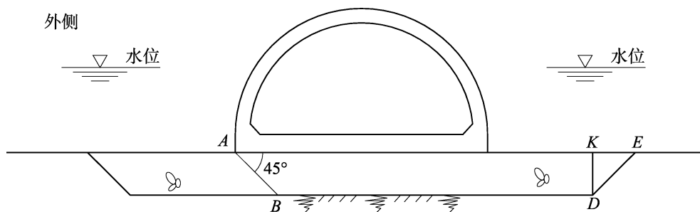
图 6.2.3-2 暗基床滑动面示意图
