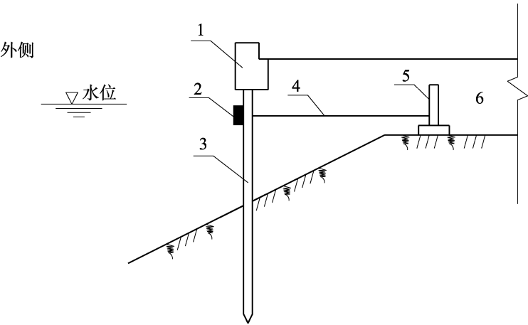
图 8.2.3 有锚板桩护岸结构断面型式 1-胸墙或帽梁;2-导梁;3-板桩;4-钢拉杆;5-锚碇结构;6-回填料
