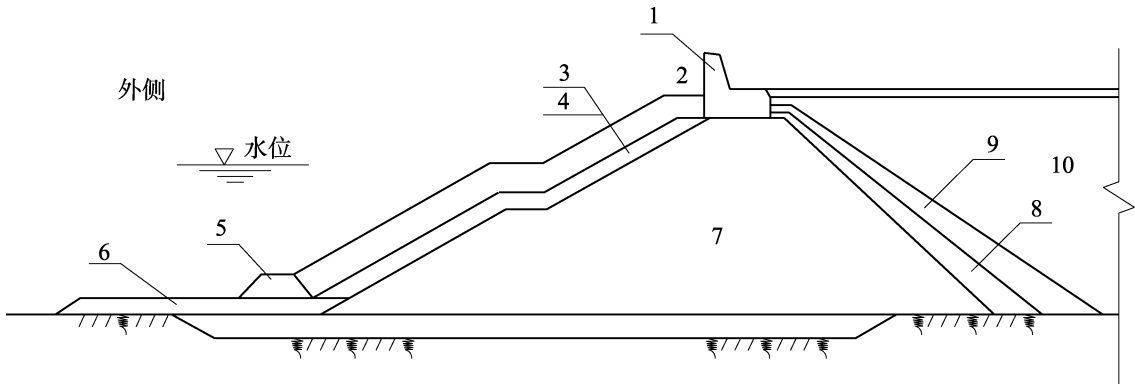
图 7.2.1-1 堤式护岸断面型式
