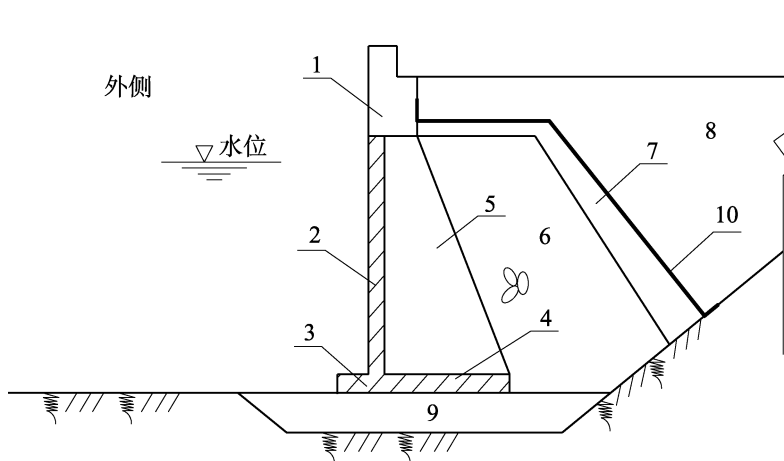
图 8.2.5 扶壁式护岸结构断面型式
