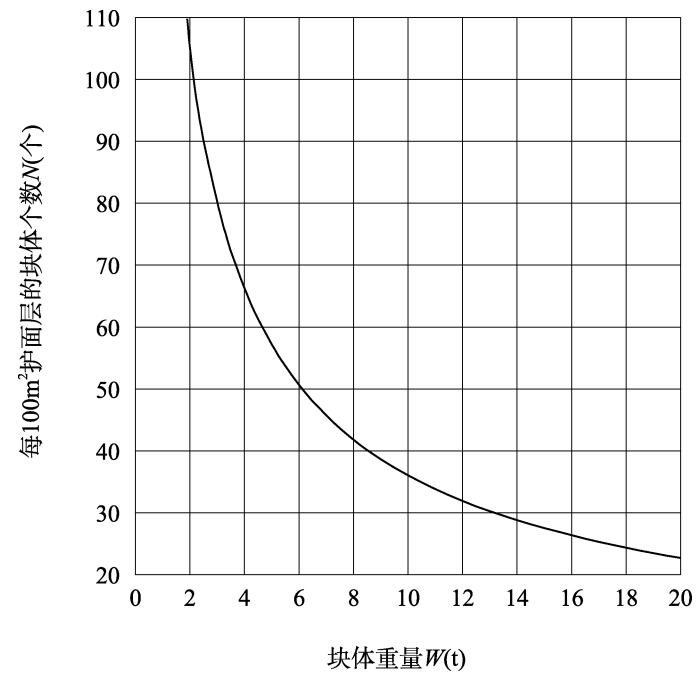
图 C.0.4-2 扭工字块体的个数 N (随机安放 2 层)
