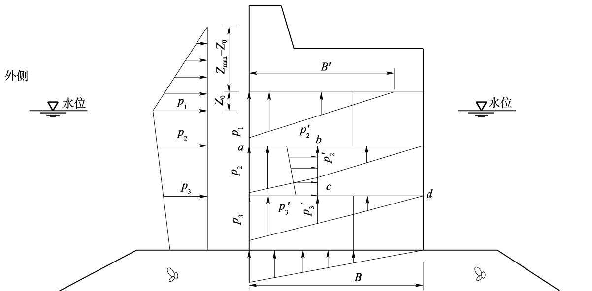
图 5.3.6 方块堤身齿缝计算示意图
