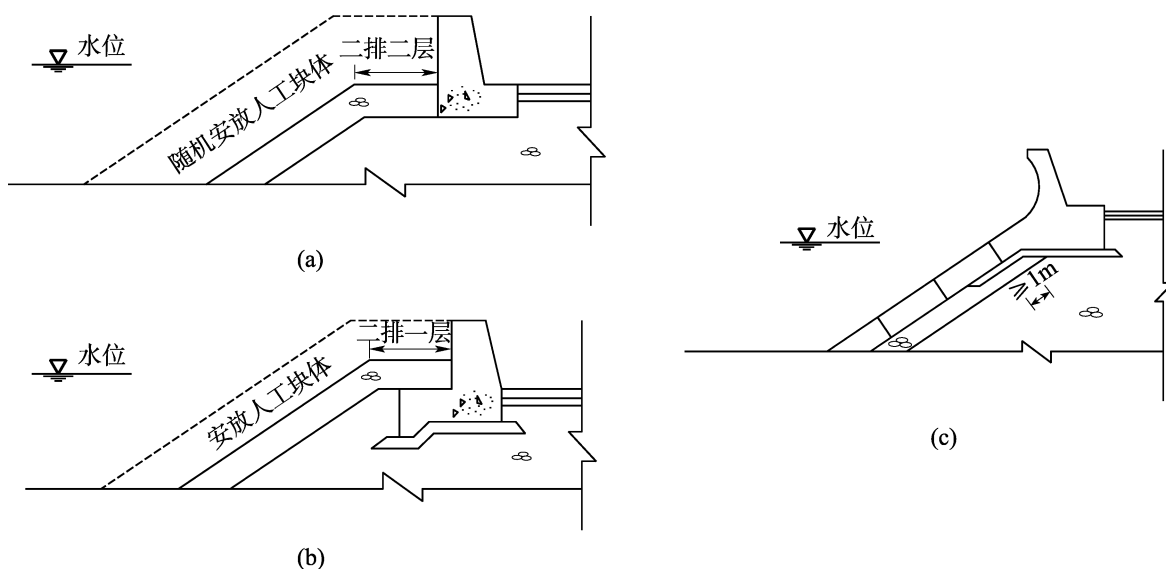
图 4.2.7 堤顶胸墙
