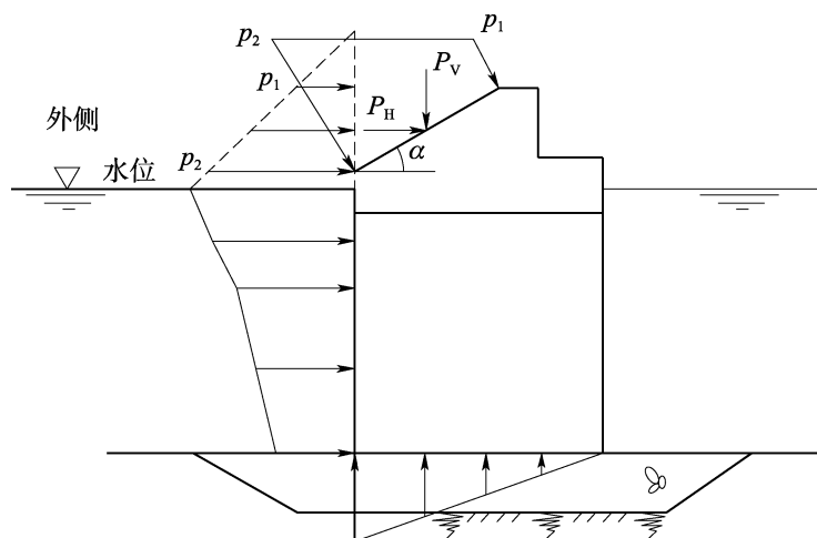
图 G.0.1 削角直立堤波压力图
