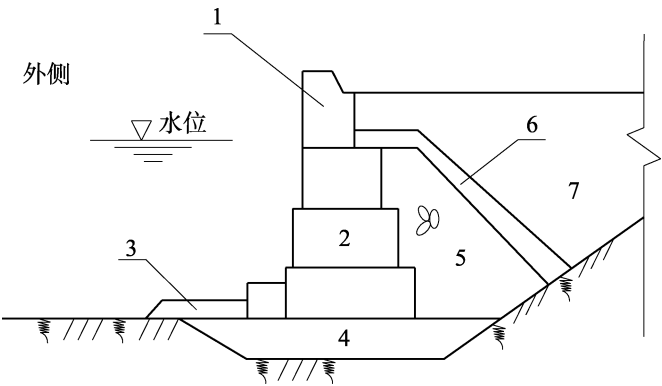
图 8.2.2 混凝土方块护岸结构断面型式 1-胸墙;2-墙体;3-护底;4-基床;5-抛石棱体;6-倒滤层;7-回填料
