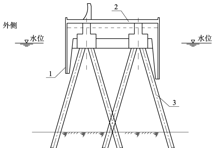
图 6.3.1 桩基透空堤断面型式
