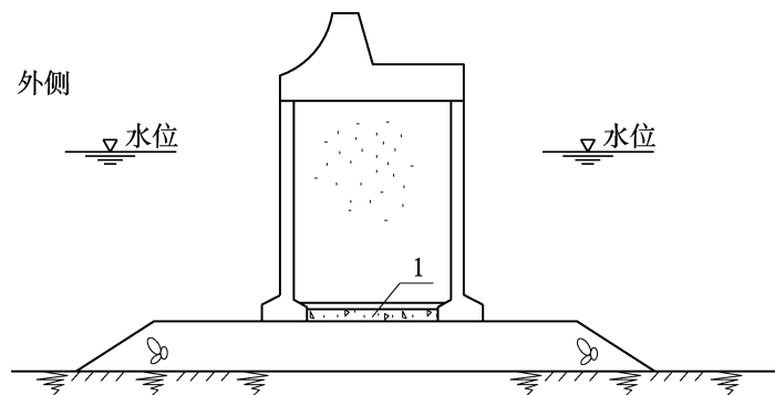
图 5.7.1 坐床式圆筒直立堤断面型式
