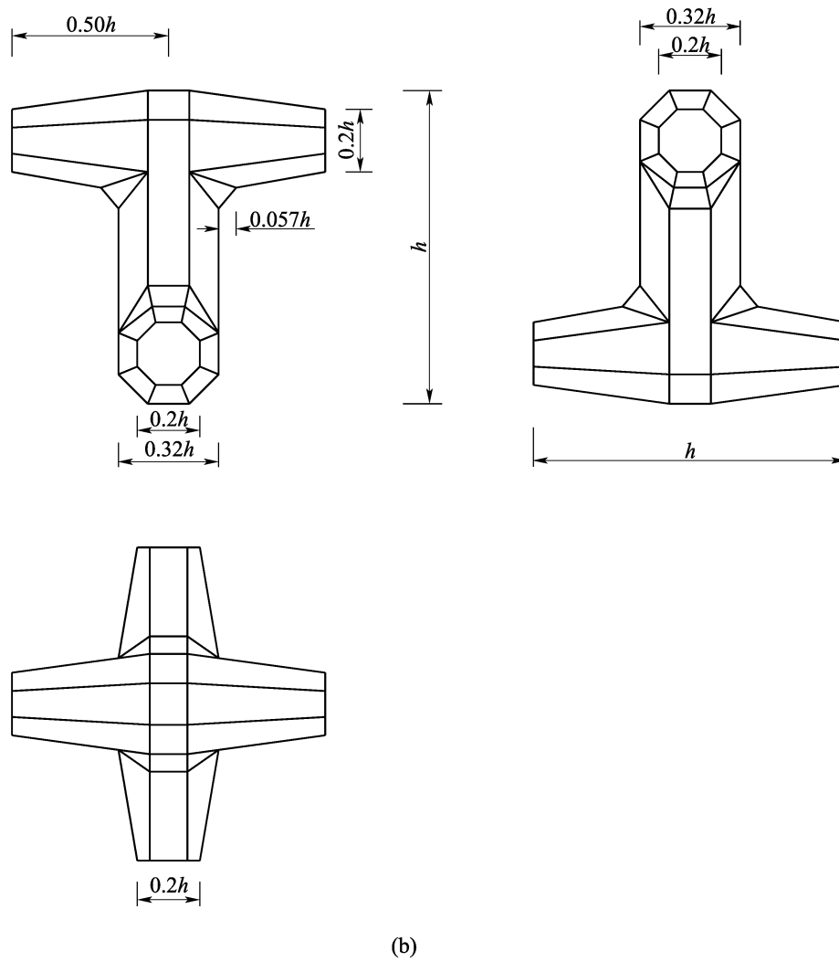
图 B.0.1-3 扭工字块体 (a) A 型扭工字块体; (b) B 型扭工字块体 h -扭工字块体正向高度
