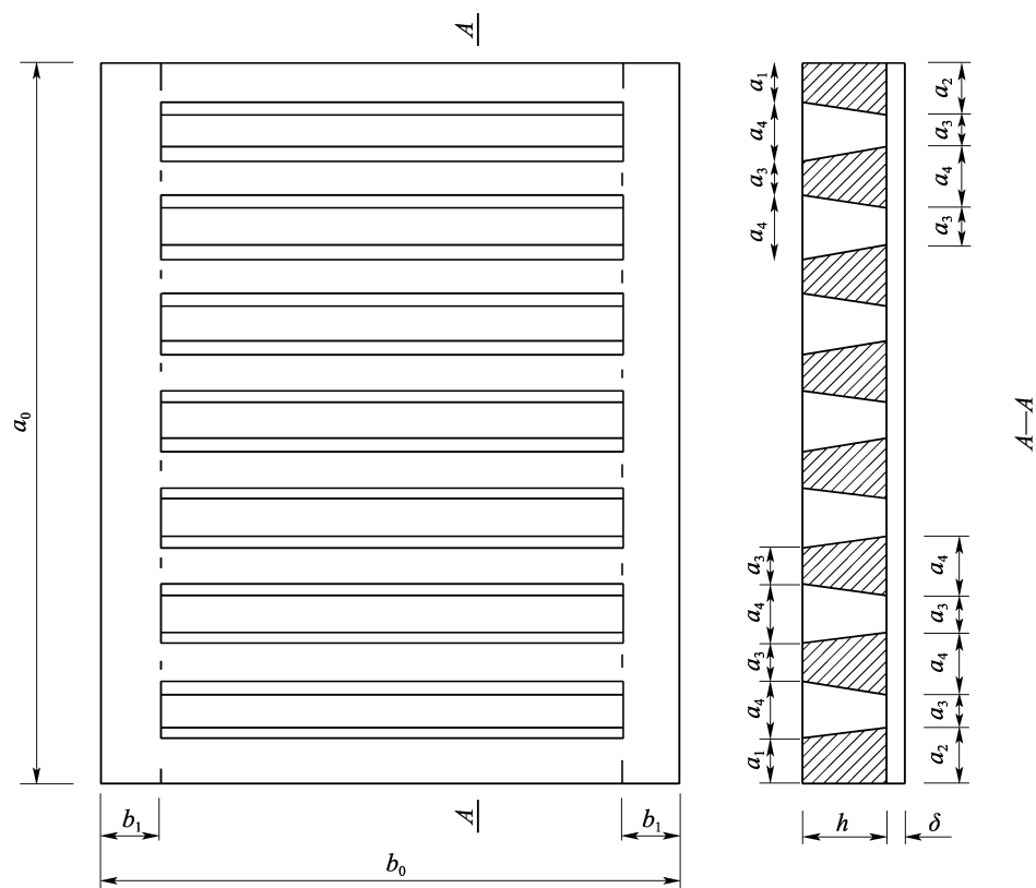
图 4.3.19 栅栏板结构图
