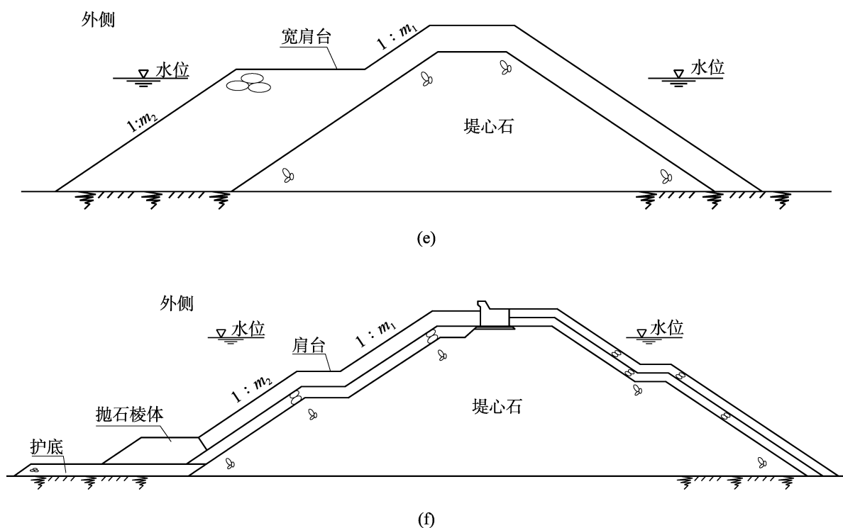
图 4.2.1 斜坡堤断面型式
