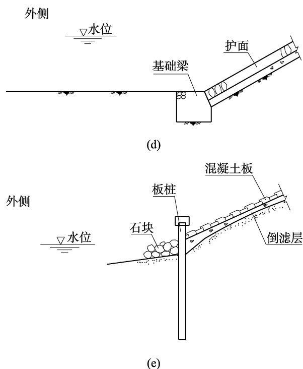
图 7.2.3 护脚结构型式
