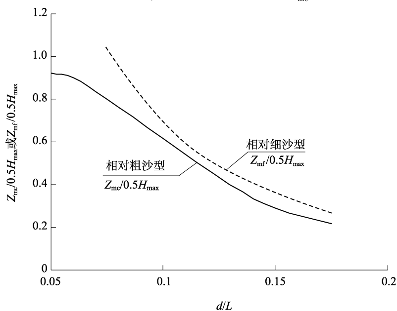
图 D.0.6 冲刷谷最大深度计算图
