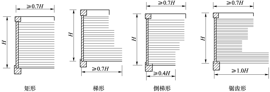
图 8.2.10 加筋土岸壁断面型式 H -岸壁高度
