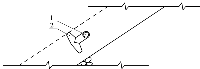
图 4.4.5-1 扭工字块体随机安放示意图
