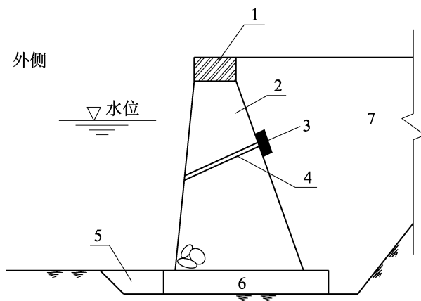
图 8.2.1 现浇混凝土或浆(灌)砌块石护岸结构断面型式 1-压顶;2-墙体;3-倒滤设施;4-排水孔;5-护底;6-底板;7-回填料
