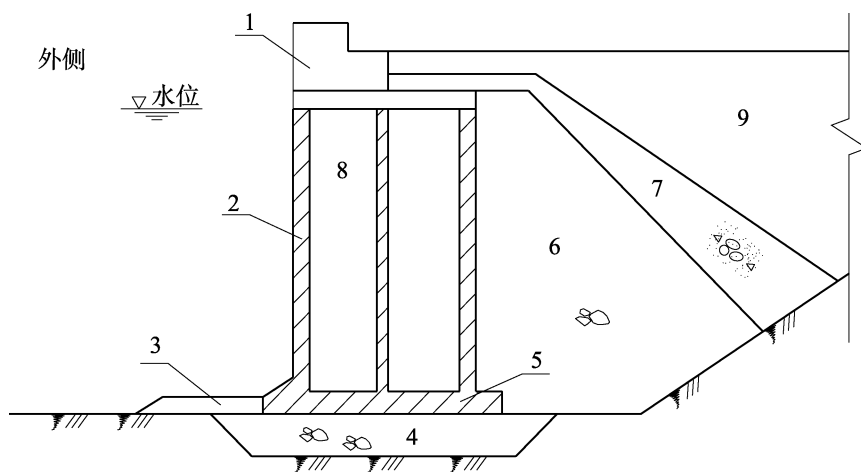
图 8.2.6 沉箱式护岸结构断面型式
