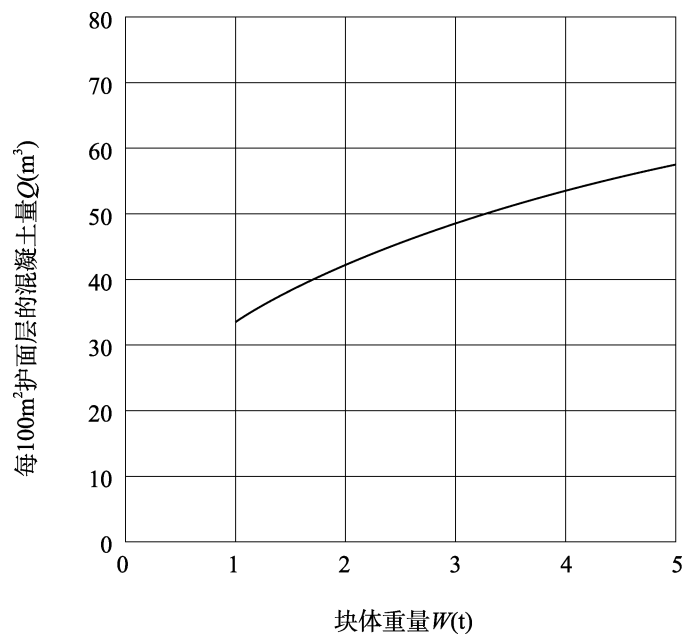
图 C.0.3-3 四脚空心方块混凝土量 Q
