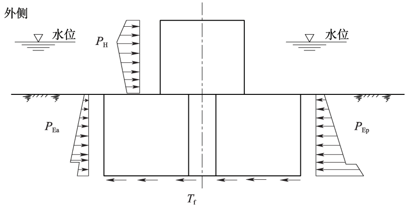
图 K.0.2 箱筒型基础结构防波堤抗滑稳定性计算简图
