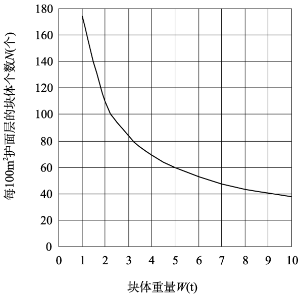
图 C.0.2-2 四脚锥体的块体个数 N
