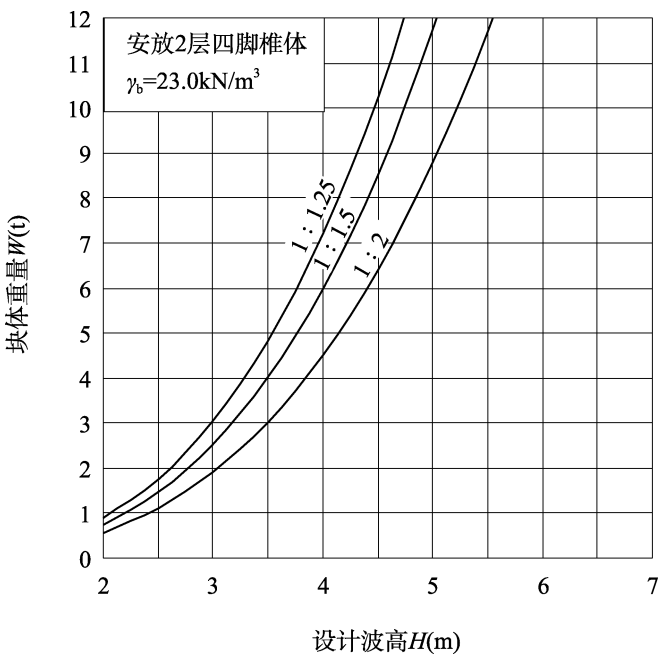
图 C.0.2-1 四脚锥体的稳定重量 W
